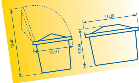
Dimensions du local technique : L x l x H = 1630 x 1210 x 1004 mm
